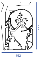
B25 plafondmontage
